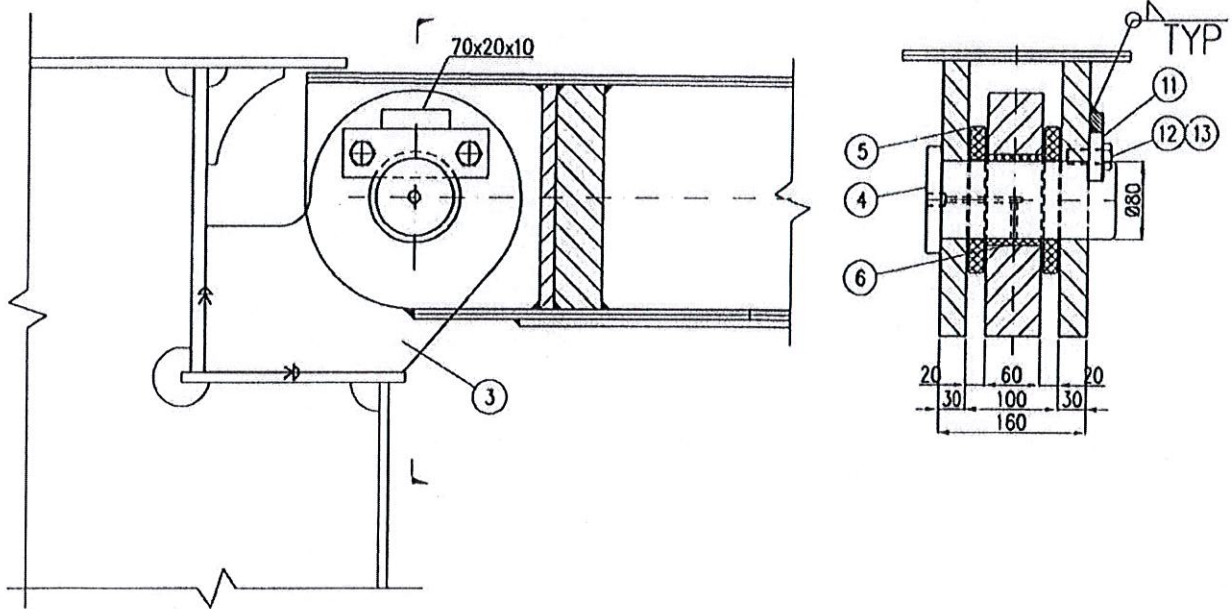
Hinge for 4480 from CL menteşeleri
