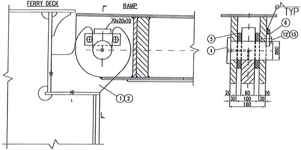
Hinge for CL ve hinge for 2240 from CL menteşeleri
